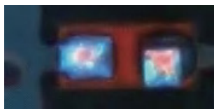
立碑 Tombstoning
